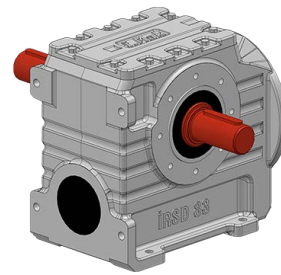
İRSD...SD Çift çıkış milli Double output shaft Double arbre de sortie
